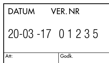
Reiner DN53A Textyta 50 x 30 mm
